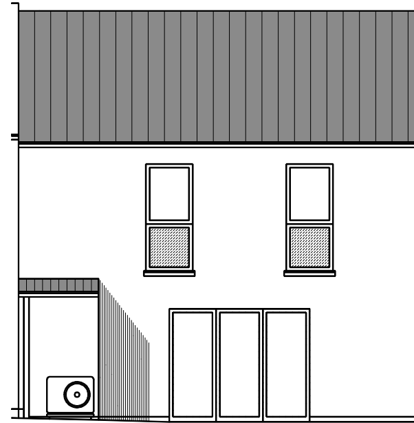
Façade Nord - M4
